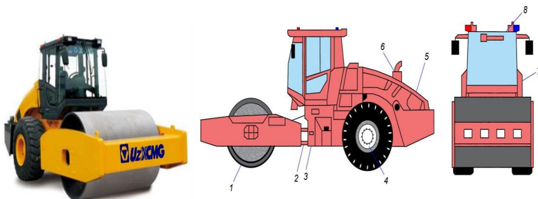
3-rasm. UzXCMG vibratsion kombinatsiyalashgan katogi .
