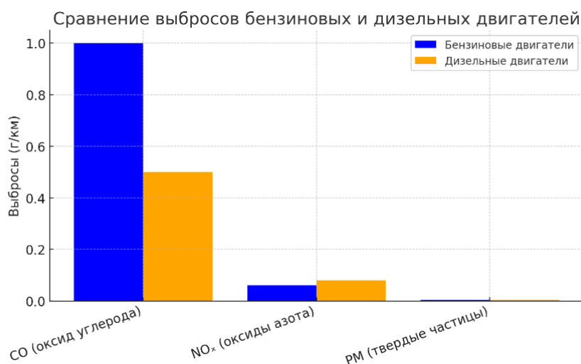
Рис. 1 Сравнение выбросов бензиновых и дизельных двигателей
