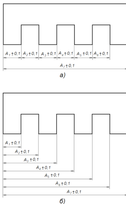
Рис.2. Способы простановки размеров детали типа гребенка:
