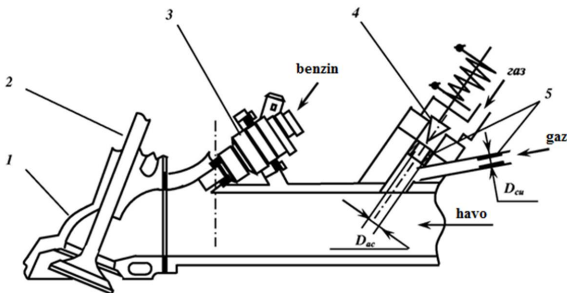
1 – kiritish quvuro'tkazgichi; 2 – kiritish klapani; 3 – benzin elektromagnit klapani; 4 – gaz elektromagnit klapani; 5 – dozalovchi unsurlar
