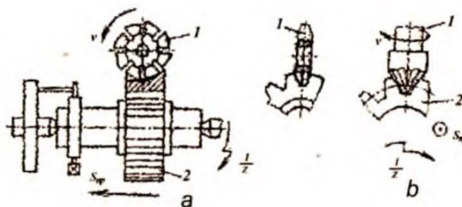
163-rasm. Tishli g'ildiraklarning tishlarini kopirlash metodida frezlash
