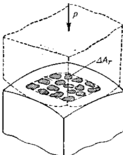
1-rasm. Metall detalning mexanik tutashishi:
