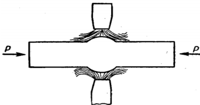
2-rasm. Bosim ostida payvandlash chizmasi.
