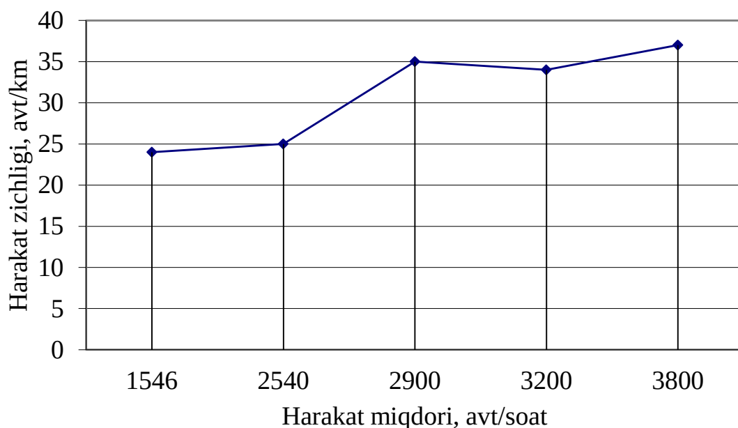
3-rasm. A.Navoiy ko'chasida harakat zichligining o'zgarishi.
