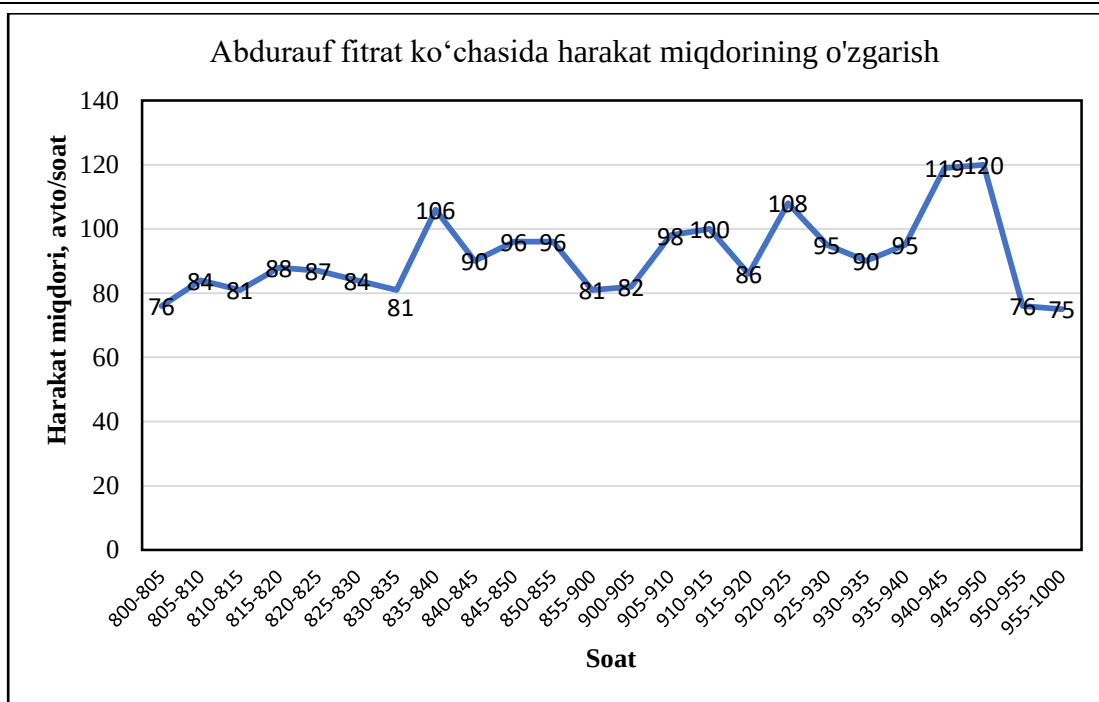
1-rasm. Transport oqimi harakat miqdorining soatlar bo'yicha o'zgarish grafigi.
