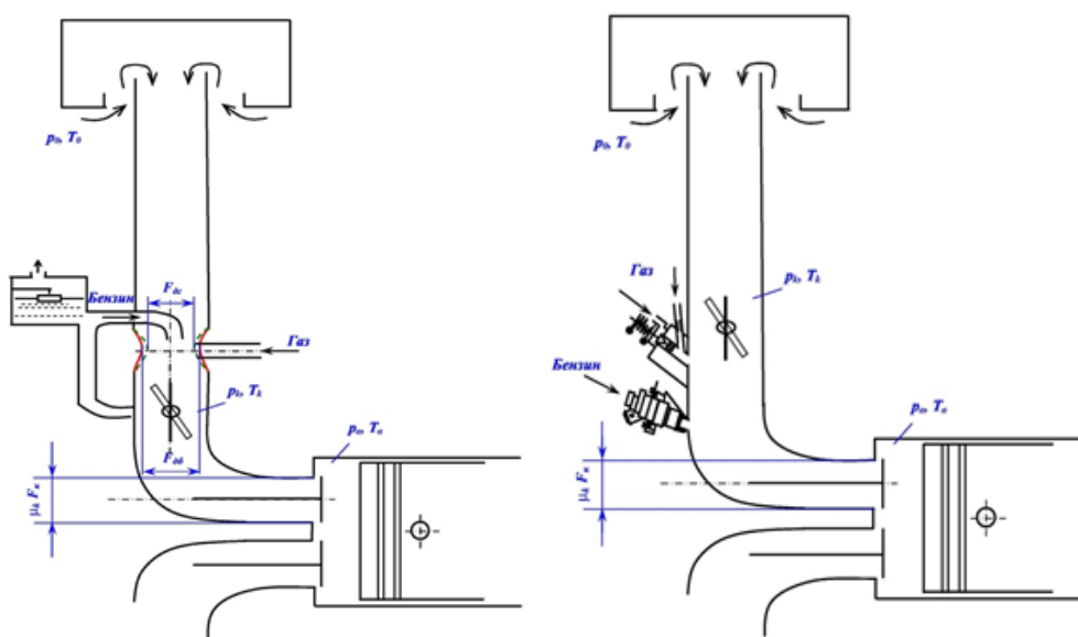
1- rasm. Ejektorli va injektorli ta’minlash tizimidagi yonilg’i (benzin yoki gaz) uzatishning sxemasi
