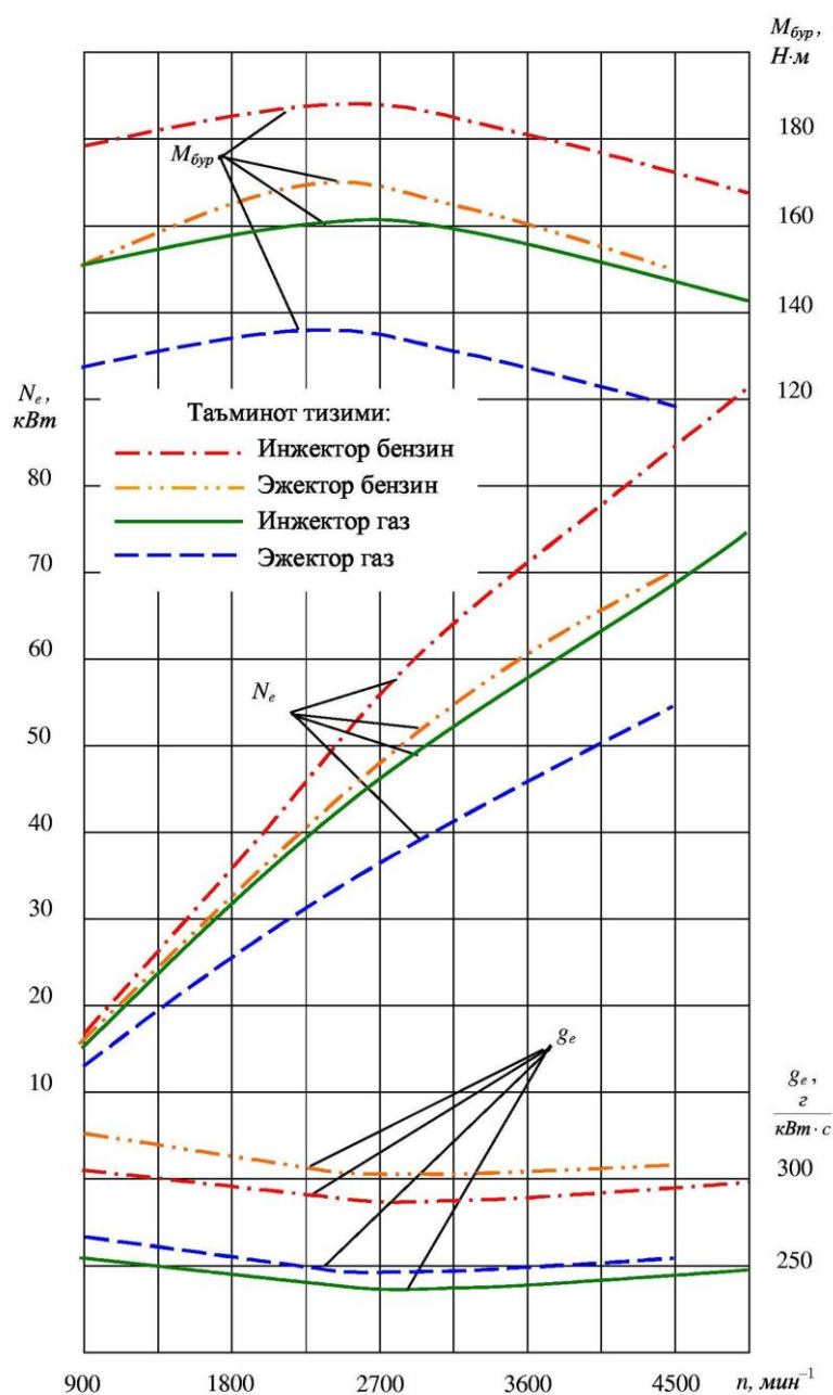
3-rasm. Turli ta'minlash tizimli V_h = 2,445 l bo'lgan to'rttaktli dvigatelning tashqi tezlik tasnifi (hisobiy)
